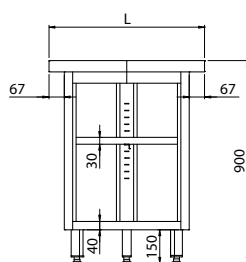
Stanowisko z szafką narożną zewnętrzną 45°
